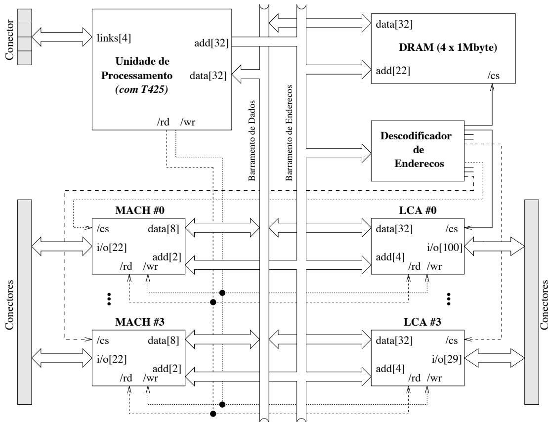
Figura 1: A arquitectura da plataforma EDgAR.
