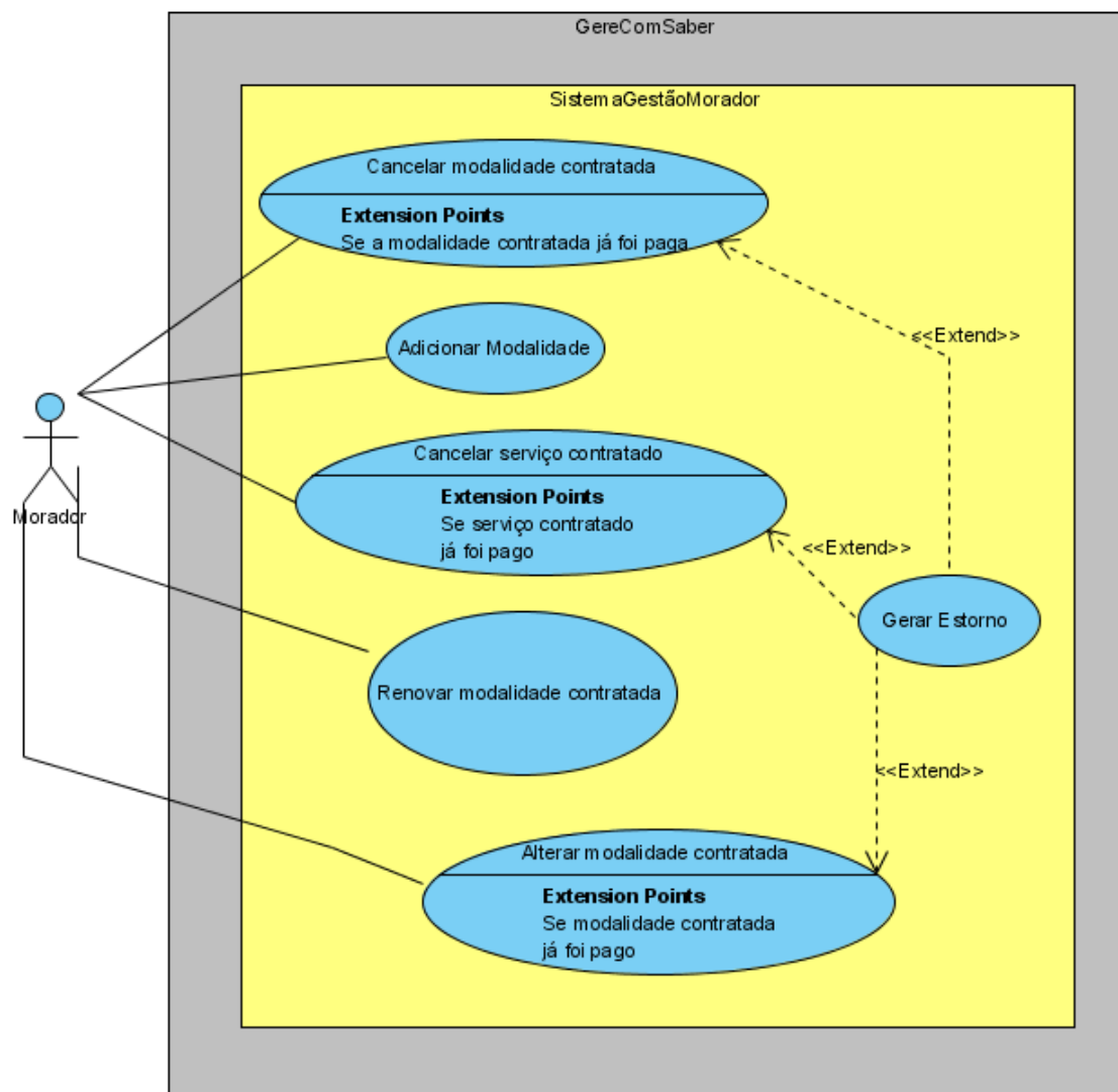
Figura 4 – Subdiagrama Atualizar Serviços Contratados
