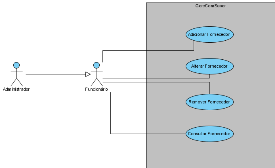
Figura 11 – Subdiagrama Gerir Fornecedores
