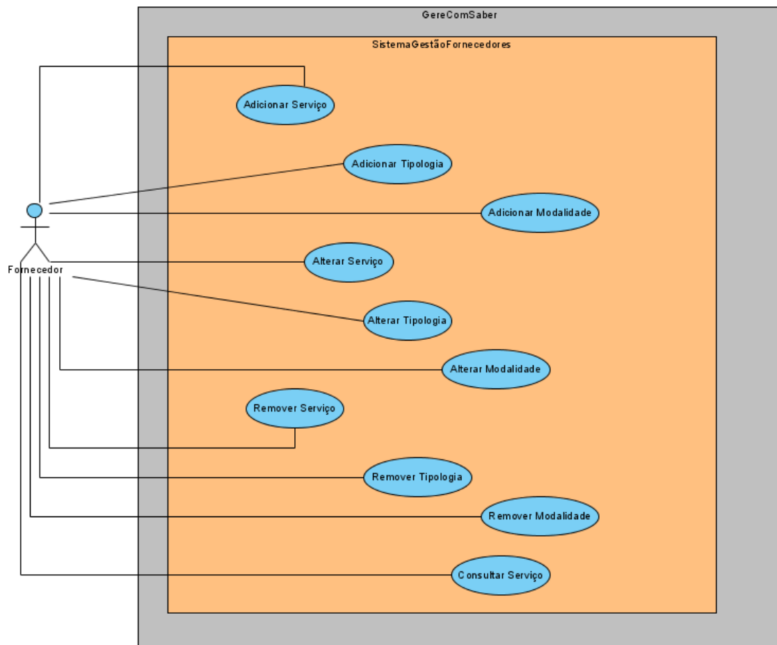
Figura 8 – Subdiagrama Gerir Serviços
