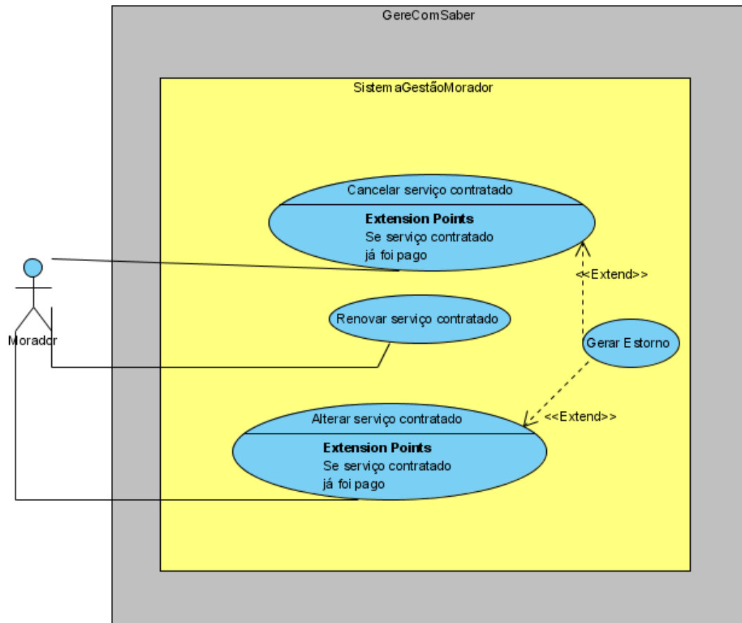
Figura 4 – Subdiagrama Atualizar Serviços Contratados
